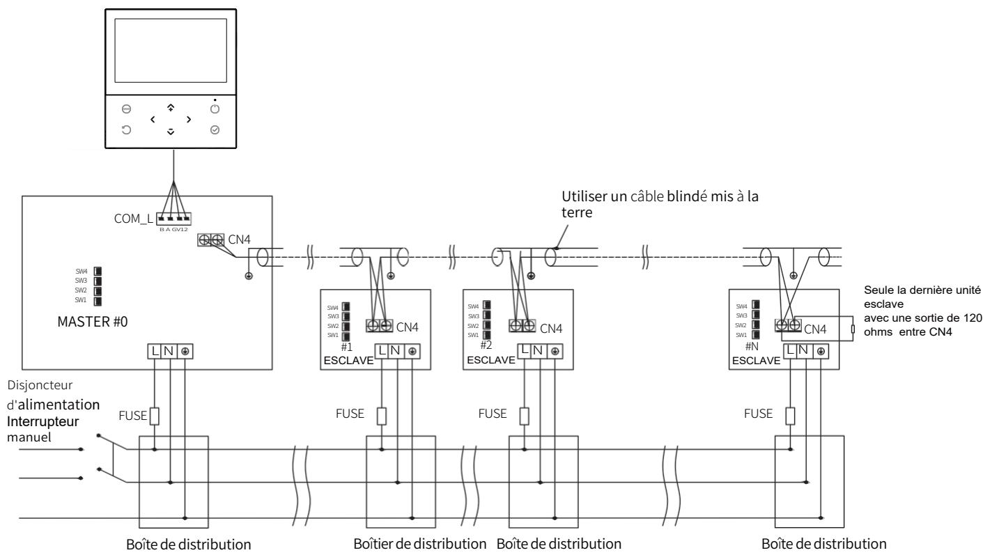
Schéma de câblage du système en cascade pour les modèles monophasés 4~16 KW
