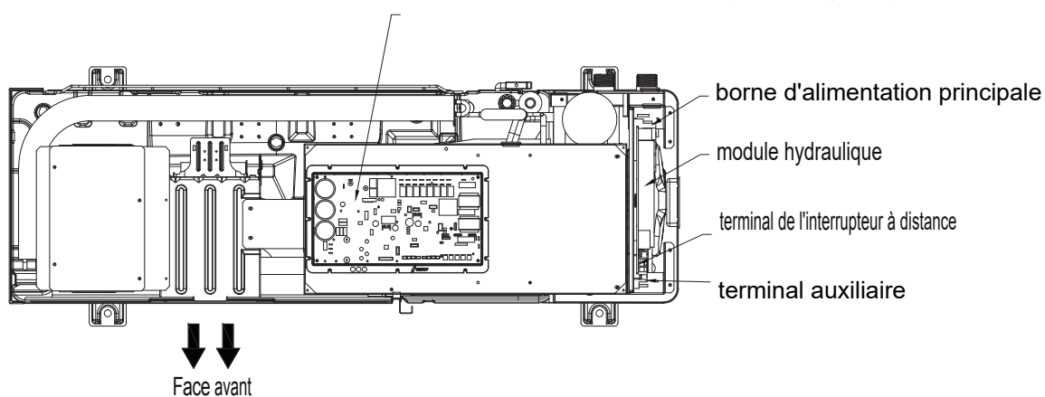
Carte de circuit imprimé de l'entraînement et du système de réfrigération (carte de circuit imprimé A)
